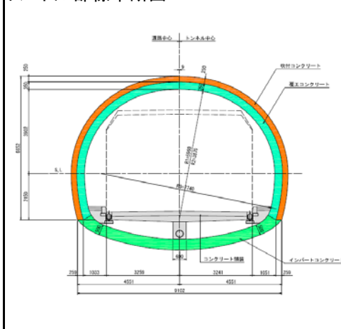
トンネル部標準断面
