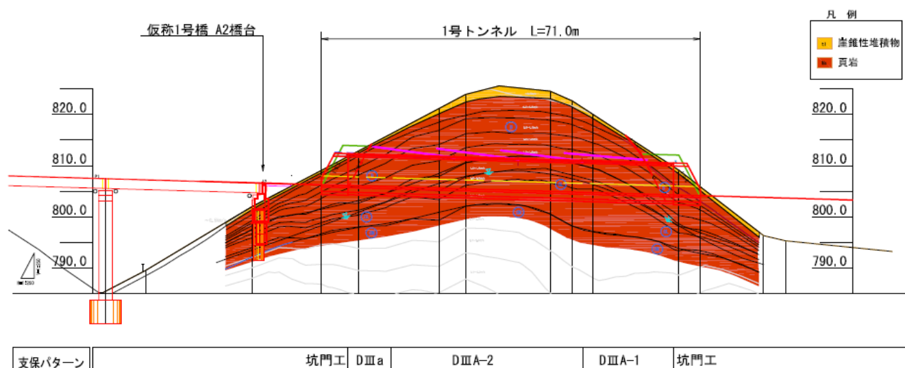
地質縦断図
