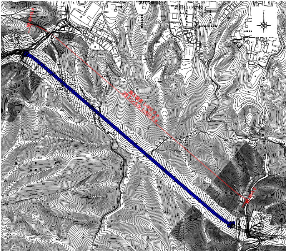
全体平面図
