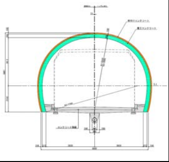
トンネル部標準断面
